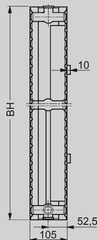
Seitenansicht Typ 21
