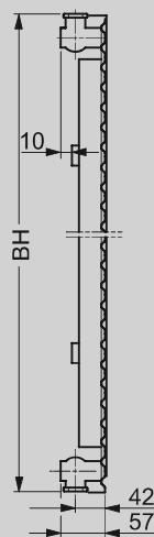
Seitenansicht Typ 20 und 22
