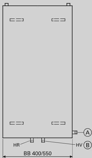
Frontansicht Typ 11, 20, 22 und 33
