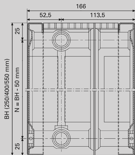
Seitenansicht Typ 33
