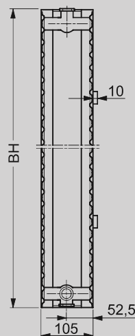
Seitenansicht Typ 33
