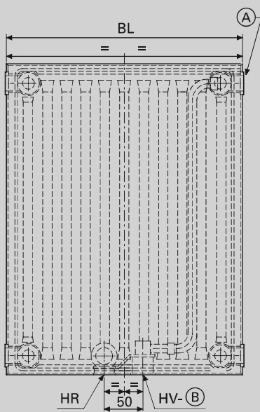
Frontansicht Typ 11, 20, 22 und 33
